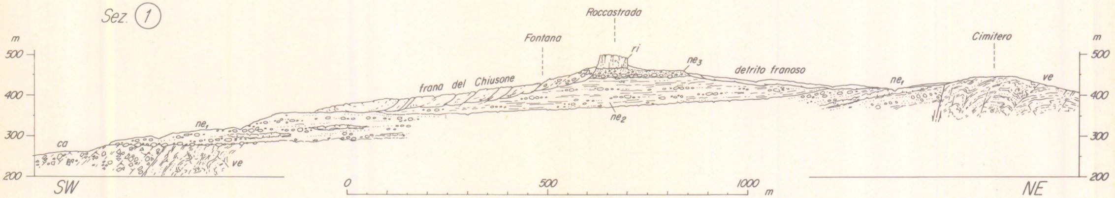
Sez. ②
