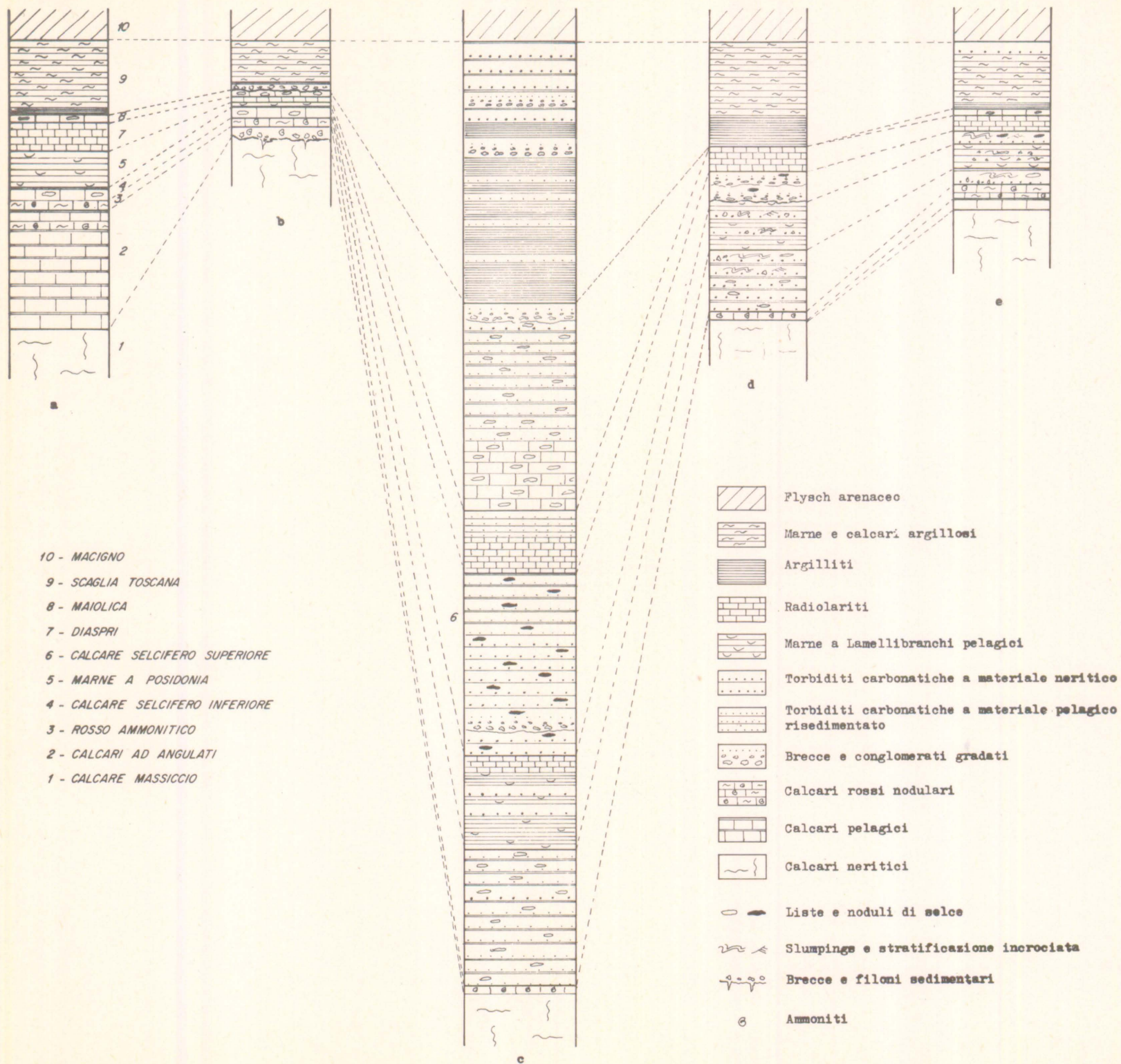
Fig. 2 - Variazioni di facies e di spessori della Serie toscana a Nord dell'Arno.
